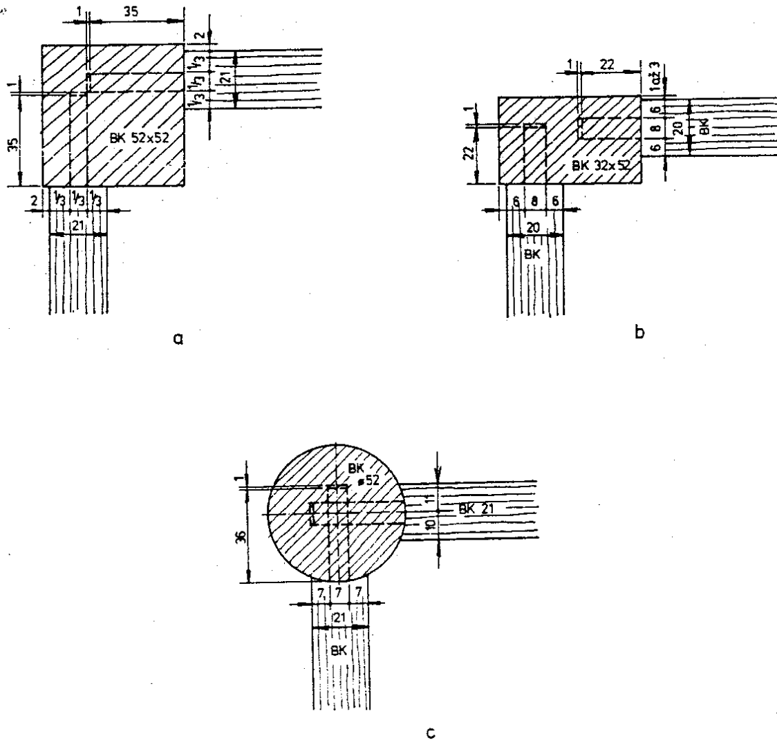
Obr. 112. Spojenie nôh s lúbmi na čap a dŕab a – štvorcová noha, b – obdĺžniková noha, c – kruhová noha
